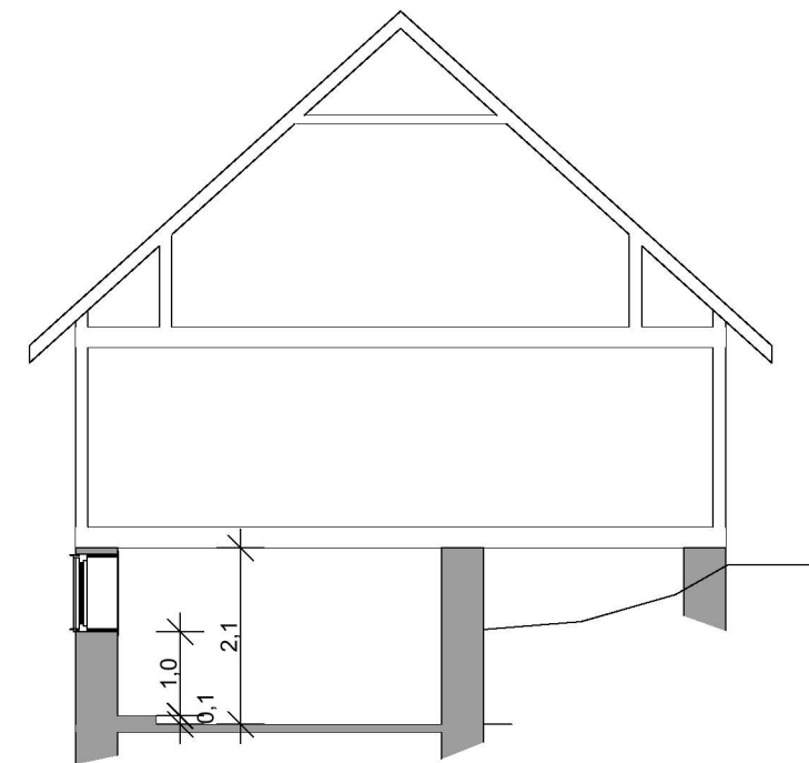
SNITT A-A
