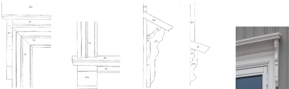
Fig.2 vindusdetaljer
